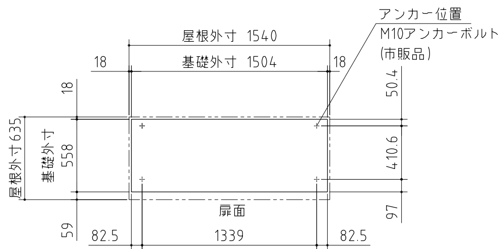
ベタ基礎図
